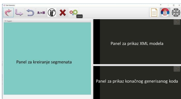
Slika 2. Grafički interfejs
